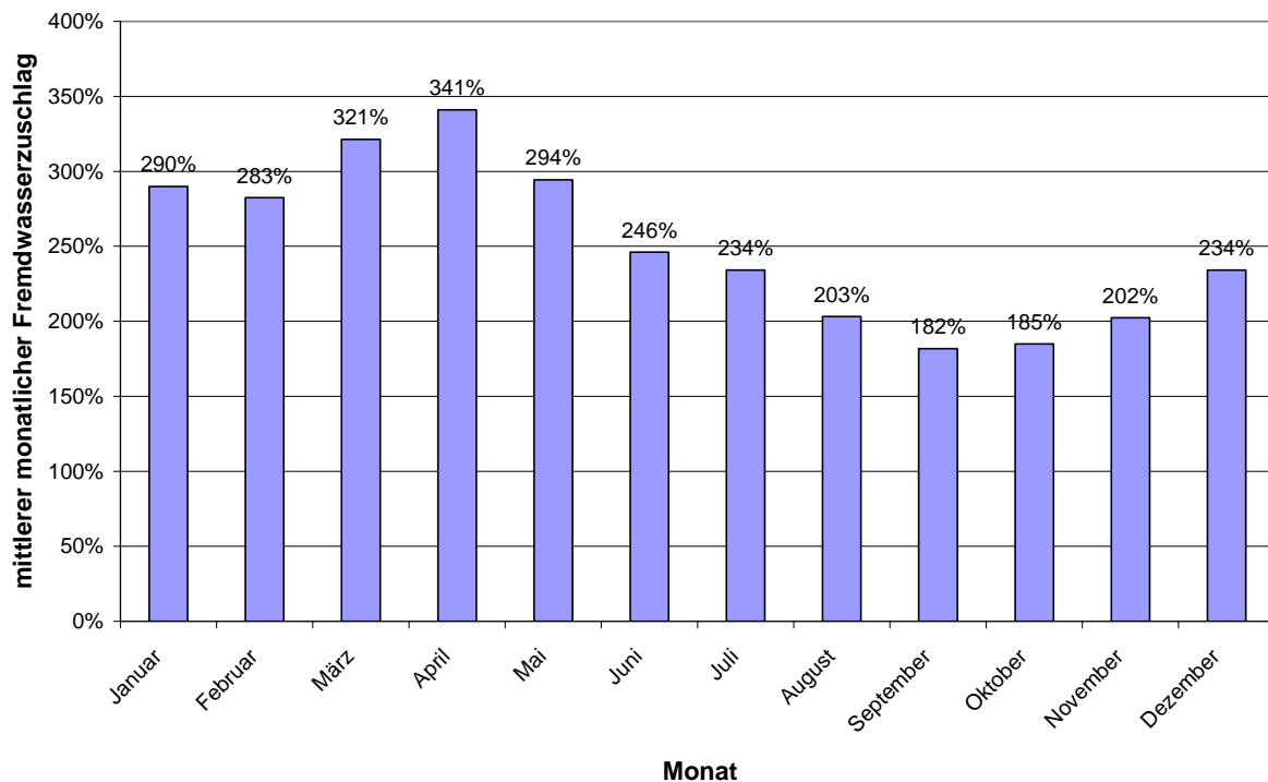
Abbildung 4-18: Mittlerer Fremdwasserzuschlag der Kläranlage Unteröwisheim berechnet nach der Methode des „gleitenden Minimums“ (monatliche Durchschnittswerte).
