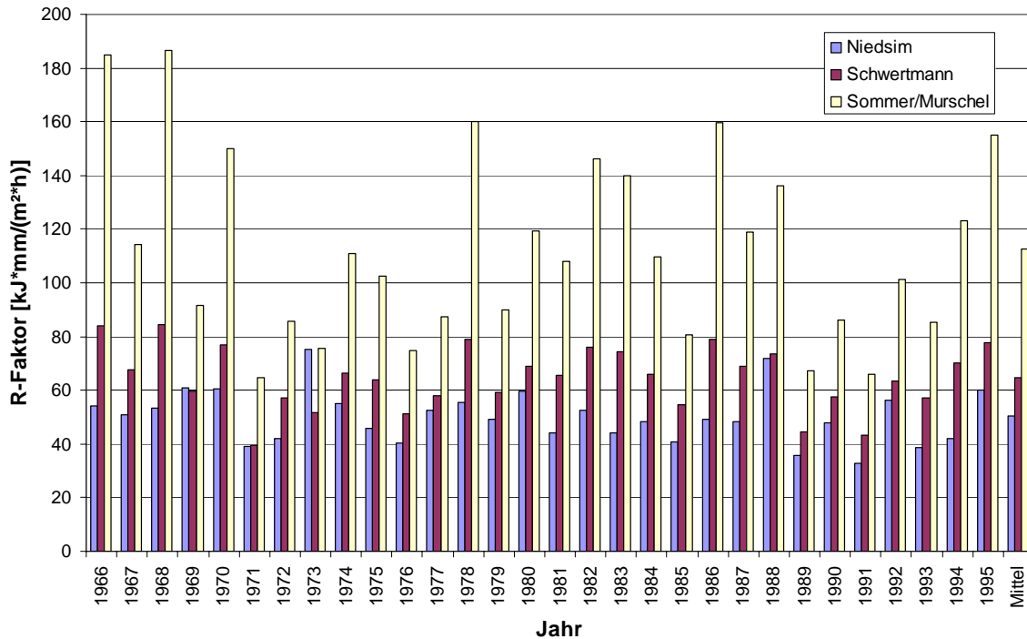
Abbildung 7-13: Vergleich der für all 30 NiedSim Jahre berechneten R-Faktoren mit den aus den Schätzformeln anderer Autoren berechneten Werten.
