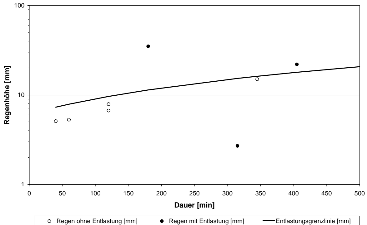
Abbildung 4-20: Zur Plausibilisierung des Kanalnetzmodells aufgestellte Entlastungsgrenzlinie des RÜB Menzingen.
