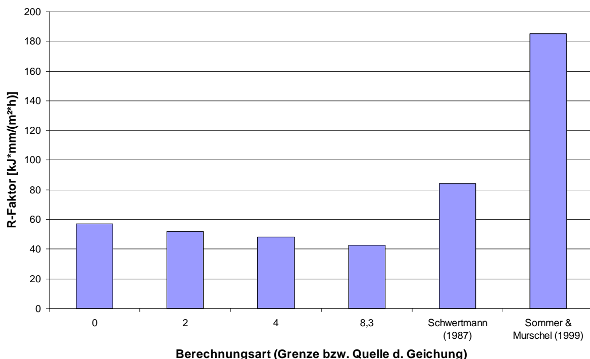
Abbildung 7-12: Vergleich der mit verschiedenen Grenzen ermittelten R-Faktoren mit den aus den Schätzformeln anderer Autoren berechneten Werten.
