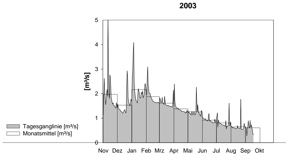
Abbildung 2-4: Tages- und Monatsmittel der Abflüsse des Jahres 2003
