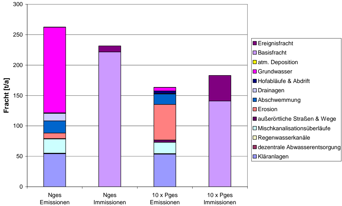
Abbildung 6-5: Emissionen und Immissionen von Stickstoff und Phosphor (10-fach überhöht): Emissionen als gestapelte, pfadspezifische Emissionen, Immissionen als gestapelte Säule aus Basisfracht und Ereignisfracht
