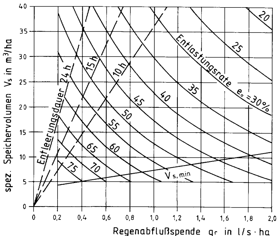
Abbildung 4-16: Spezifisches Speichervolumen in Abhängigkeit von der Regenabflusspende und der zulässigen Entlastungsrate (aus: ATV, 1992)
