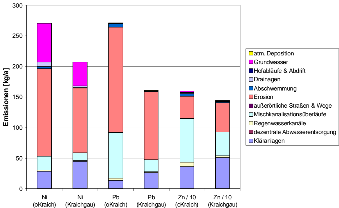
Abbildung 6-3: Summe der Emissionen für Cadmium (100-fach überhöht), Chrom, Kupfer [oben], Nickel, Blei und Zink (auf ein Zehntel reduziert) [unten] für das Gebiet des oberen Kraichbachs: In diesem Projekt berechnet (oKraich) und nach FUCHS et al. (2003) (Kraichgau)
