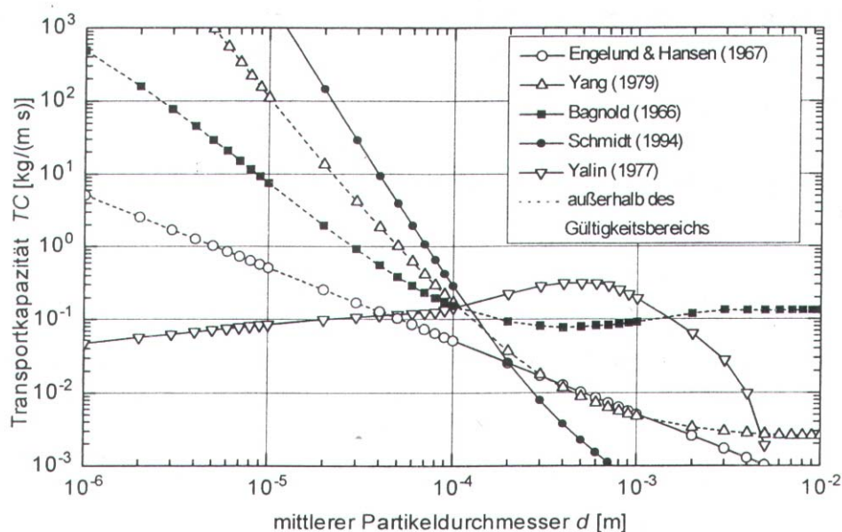
Abbildung 7-1: Korngößenspezifische Transportkapazitäten unter verschiedenen Modellierungsansätzen (GERLINGER, 1997)
