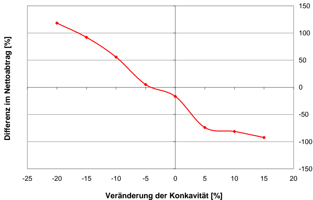
Abbildung 4-11: Abweichung des Nettobodenabtrags des Repräsentanzhanges von dem des konkaven Hanges bei Veränderung der Konkavität 13 (verändert nach SCHMITZ, 2004)
