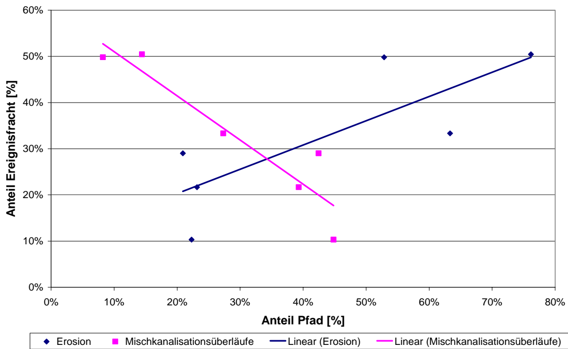
Abbildung 6-9: Anteil, den die „Ereignisfracht“ an den gesamten Immissionen hat, über dem Anteil, den der Pfad „Erosion“ bzw. „Mischkanalisationsüberläufe“ an den gesamten Emissionen hat (Schwermetalle)
