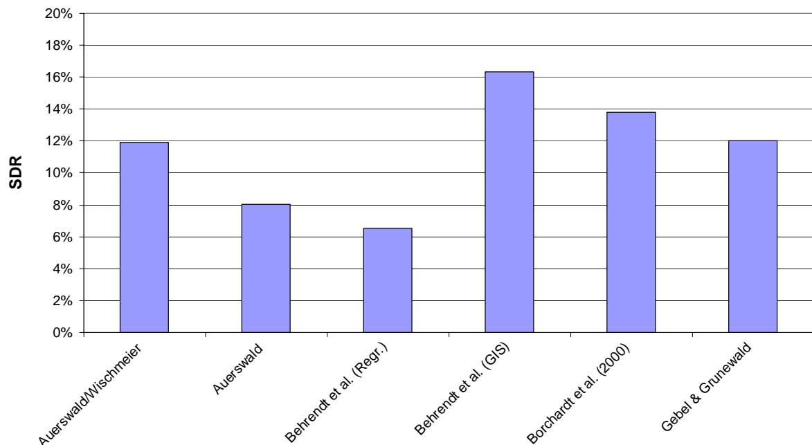
Abbildung 4-10: Für das obere Kraichbachgebiet nach verschiedenen Ansätzen (siehe Text) berechnetes Sediment-Eintragsverhältnis
