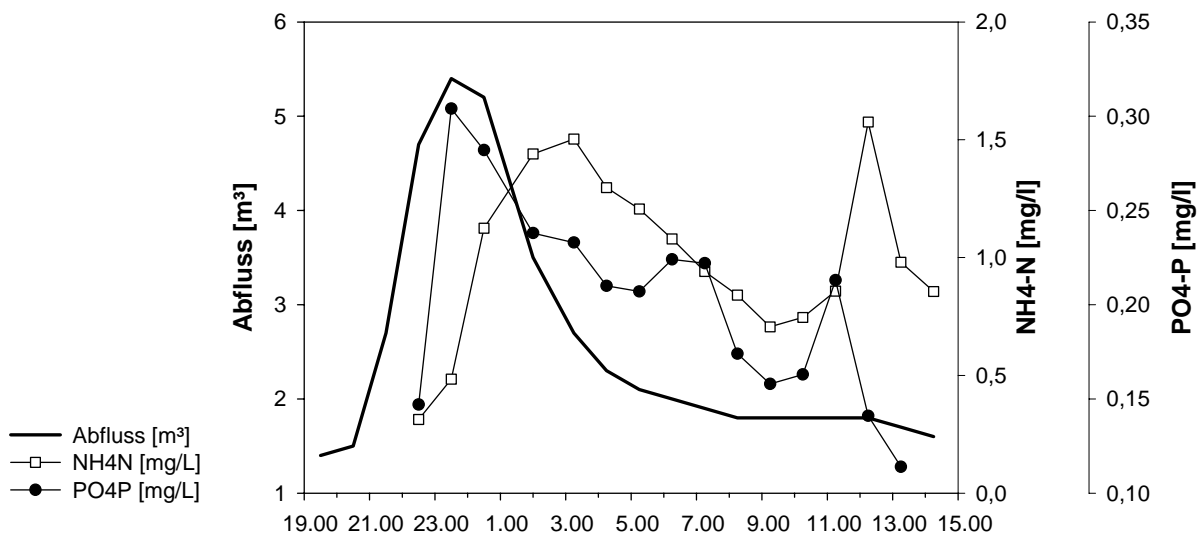
Abbildung 7-8: Phosphat-, Ammonium- und Nitritmessungen am Pegel Ubstadt während einer Abflusswelle am 30./31.03.2003
