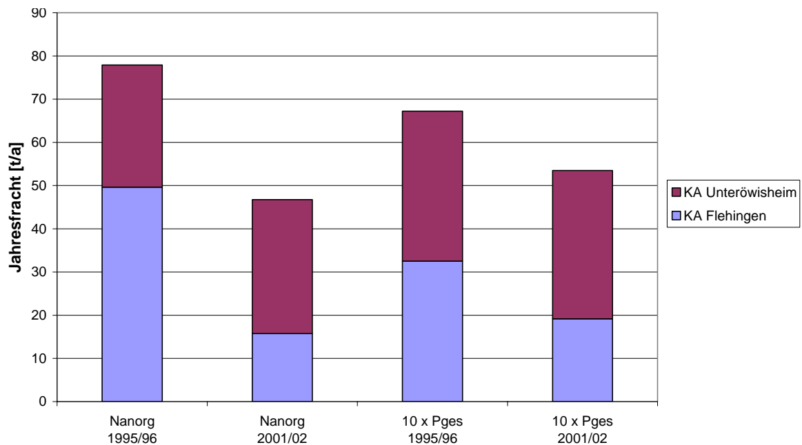
Abbildung 5-13. Nährstoffemissionen E_{KA,N,P} aus den kommunalen Kläranlagen im Einzugsgebiet des oberen Kraichbachs in den Jahren 1995/96 bzw. 2001/02
